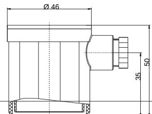
6371 IP 54 / 6372 IP 65
