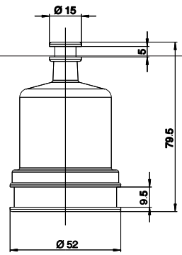
6365 IP 54
