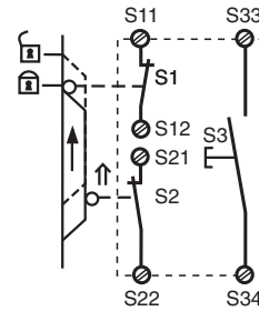
Fig. 4: Supervisión de puerta protectora bicanal, rearme manual/Comando porta di sicurezza bicanale, start manuale/Tweekanalig hekbewaking, handmatige start
