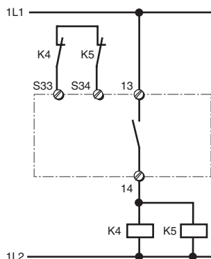
Fig. 6: Conexión de contactores externos, monocal/Esempio di collegamento per relè esterni, monocale/Aansluitvoorbeeld van externe magneetschakelaars, eenkanalig
