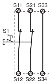
Fig. 3: Solo PNOZ X2.1: rearme automatico/Solo PNOZ X2.1: Start automat./Alleen bij PNOZ X2.1: automat. start
